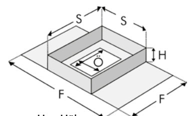
H = Höhe S = Schacht-Aussenmass F = Flansch Ö = Öffnungsmass
