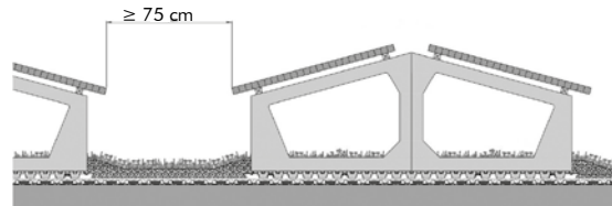
Solaraufständerung „Sattel“
